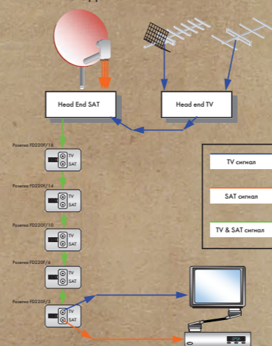
ПРИМЕР ИСПОЛЬЗОВАНИЯ РОЗЕТКИ FD220F ДЛЯ СОЗДАНИЯ „ПРОХОДНОЙ“ СЕТИ ТВ/СПУТНИК С ОДНИМ КАБЕЛЕМ IF-IF
